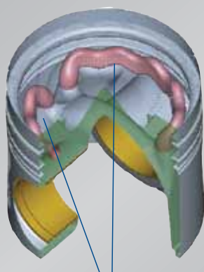
Масляный канал
